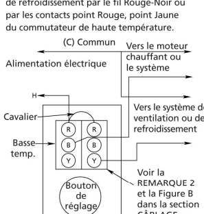
Figure 8 – Séquence de fonctionnement des thermostats SPDT/SPDT à deux étages
