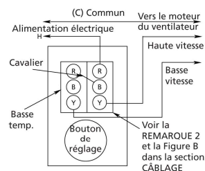
Figure 5 – Thermostats SPDT/SPDT à deux étages contrôlant un ventilateur à vitesse unique et un moteur de registre à augmentation de volume
