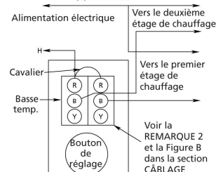
Figure 9 – Thermostats SPDT/SPDT contrôlant un système de chauffage à deux étages
