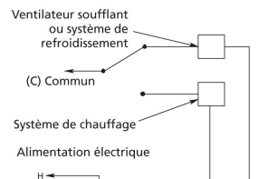
Figure 3 – Thermostats SPDT dans les systèmes de commande de chauffage et de ventilation
